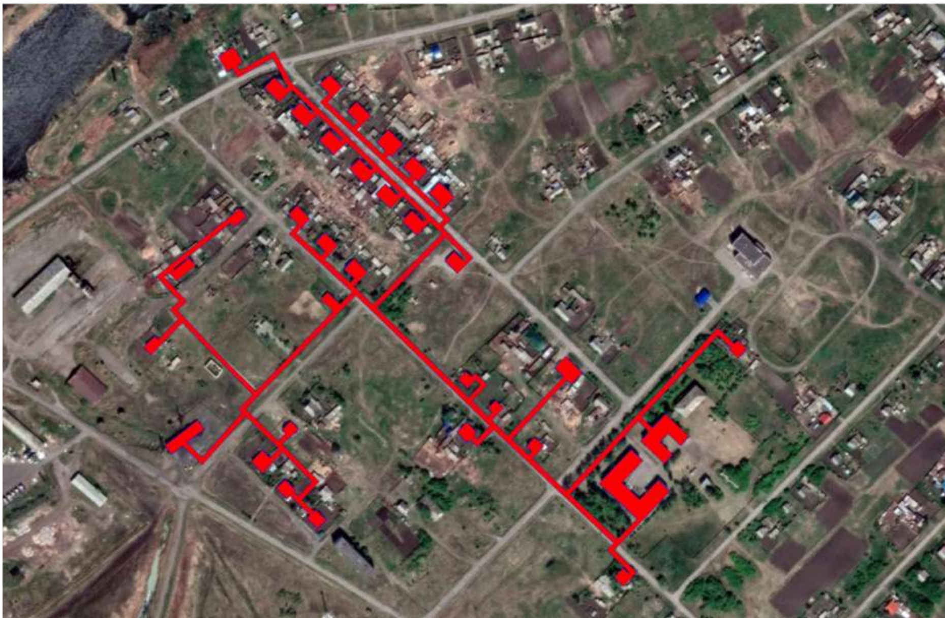
Рисунок 1.1 – Существующие и перспективные зоны действия источников теплоснабжения на территории поселка Большаковка
